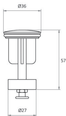
Tappo per scarico in ottone 1". Plug pop-up waste in brass 1".
