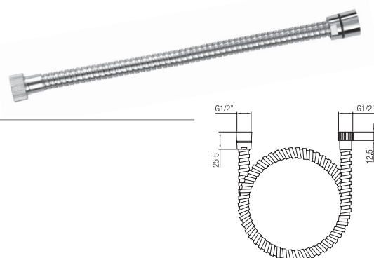
Flessibile doccia ottone conico 200 cm. Conic brass flexible hose 200 cm.
